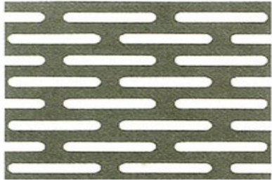
20 2.5x20 .098"x.787" -23.6% 開孔率
